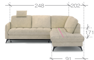
narożnik > corner sofa
